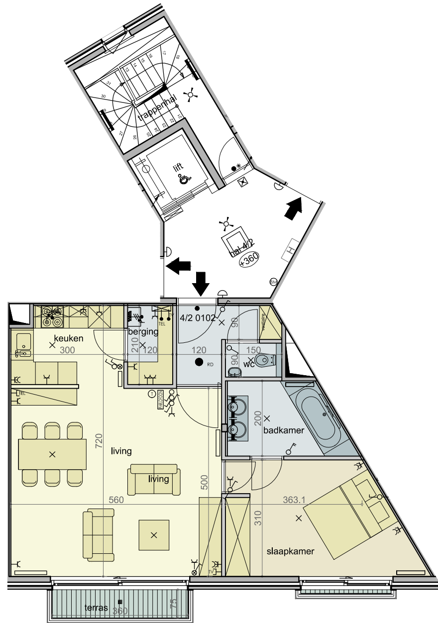
1e verdieping appartement 4/2 0102, schaal 1/100
